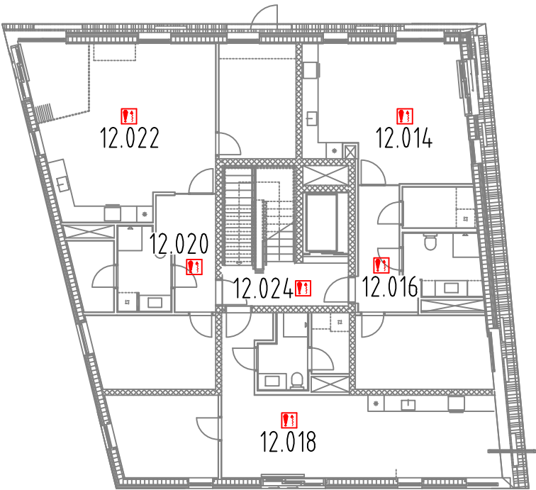
2.ETASJE
