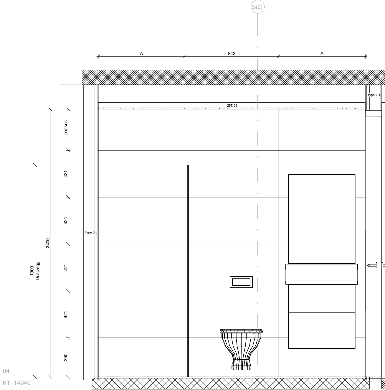
Bad 24.305 Vest 1 : 20
