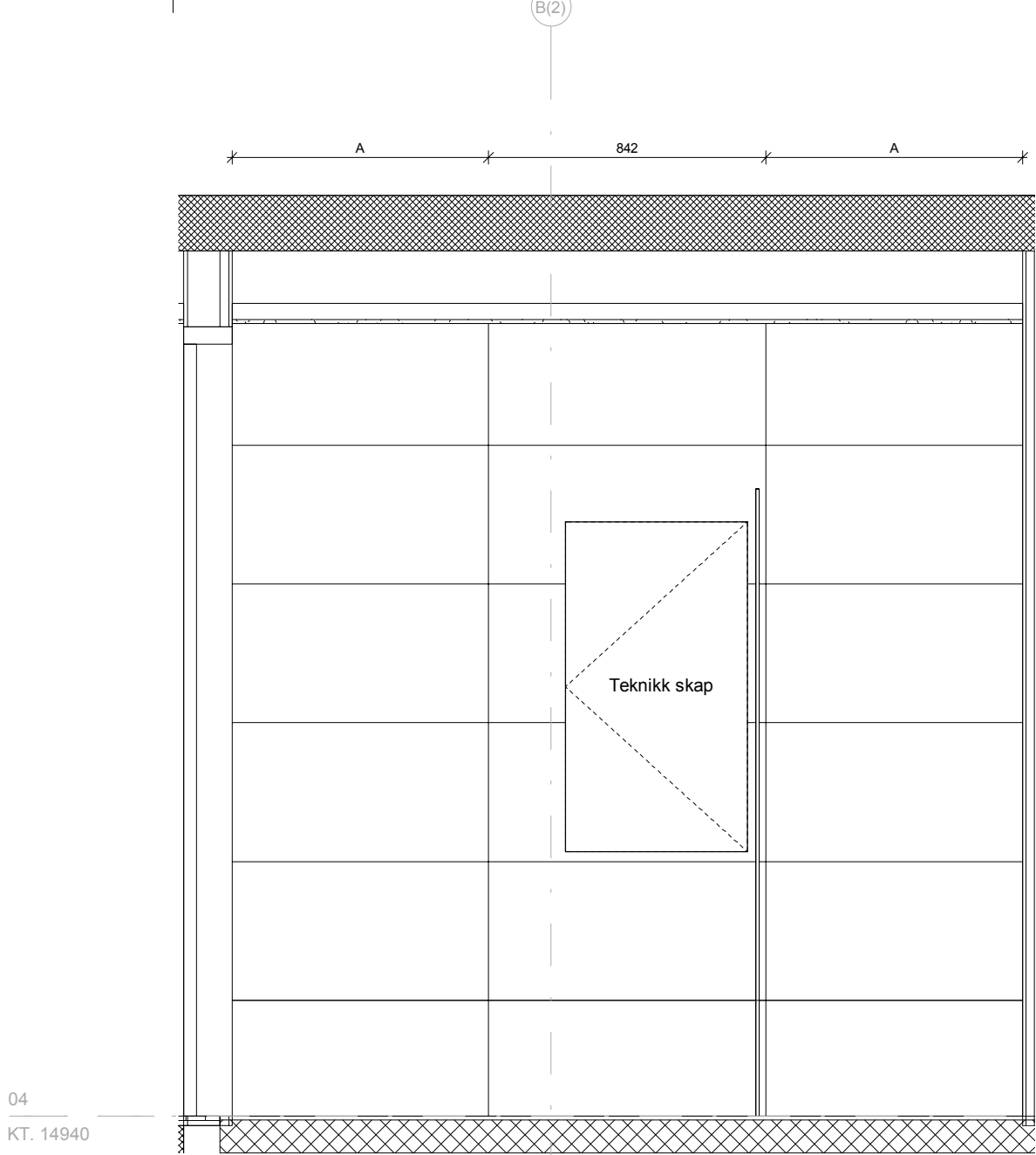
Bad 24.305 Øst 1 : 20
