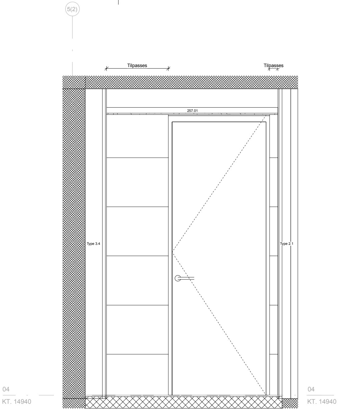
Bad 24.305 Nord 1 : 20
