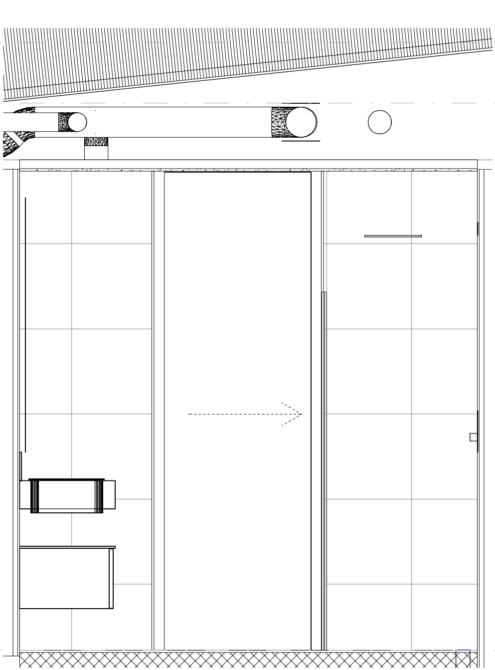
Bad 34.218 Sør 1 : 20
