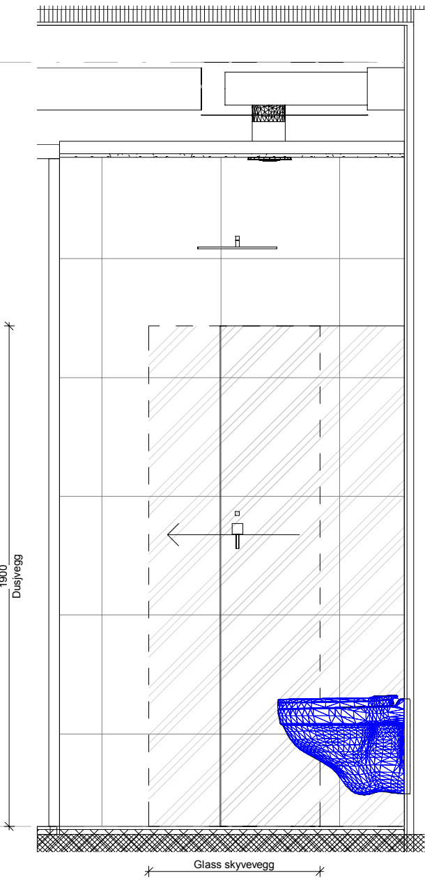
Bad 34.218 vest 1 : 20
