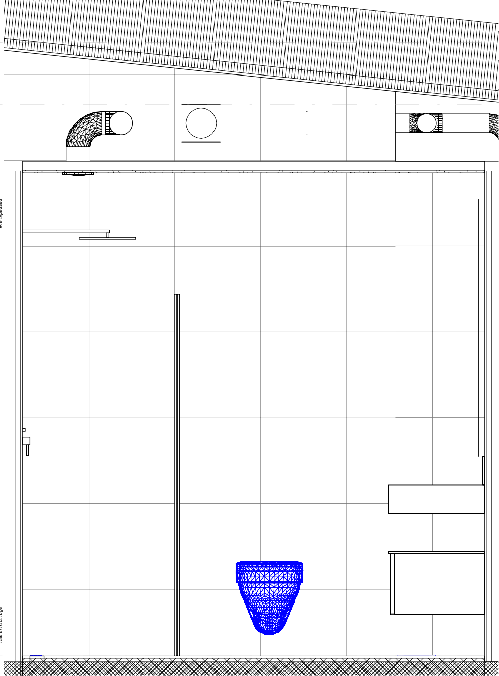
Bad 34.218 Nord 1 : 20
