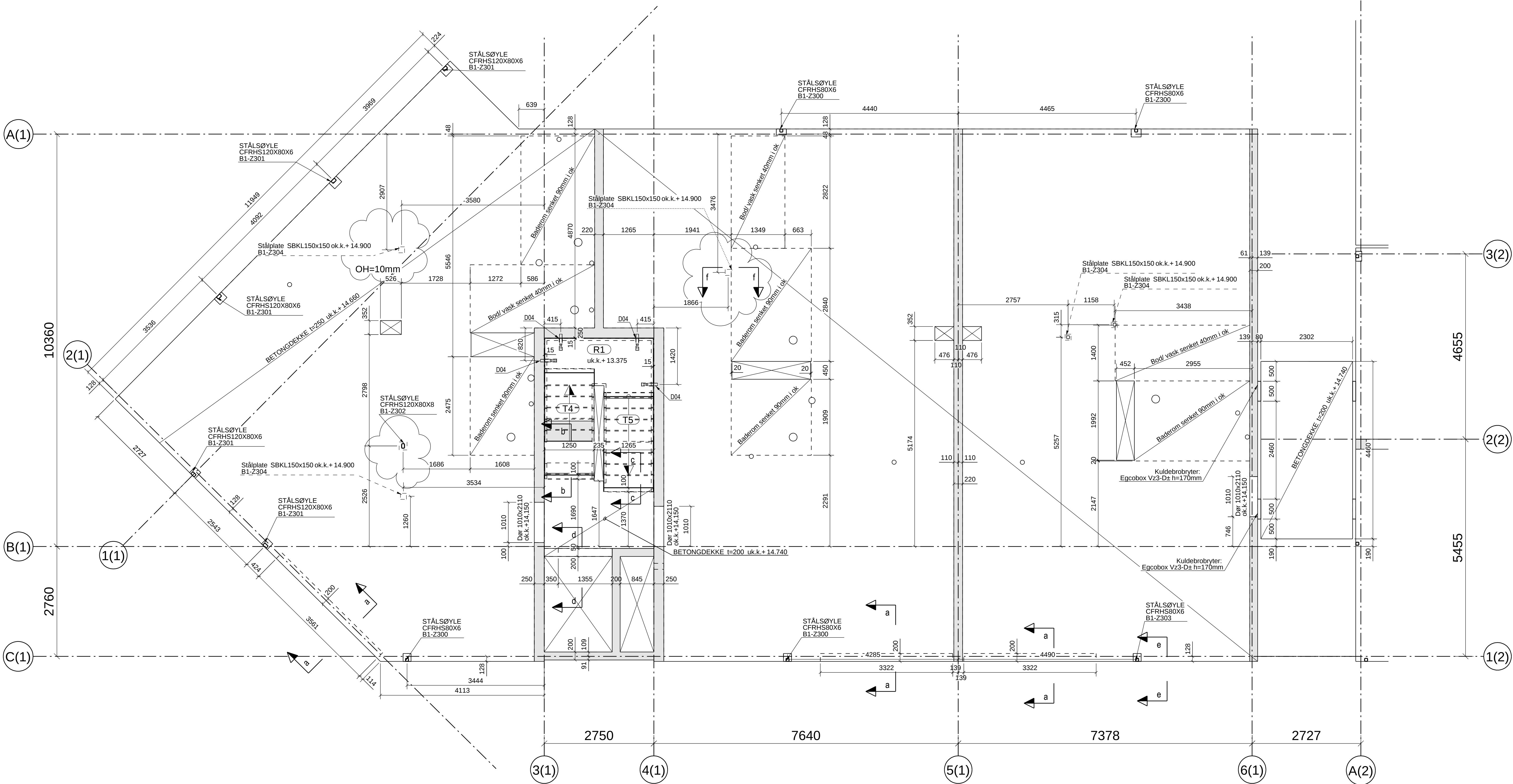
Bygg 1 PLAN +14.94
