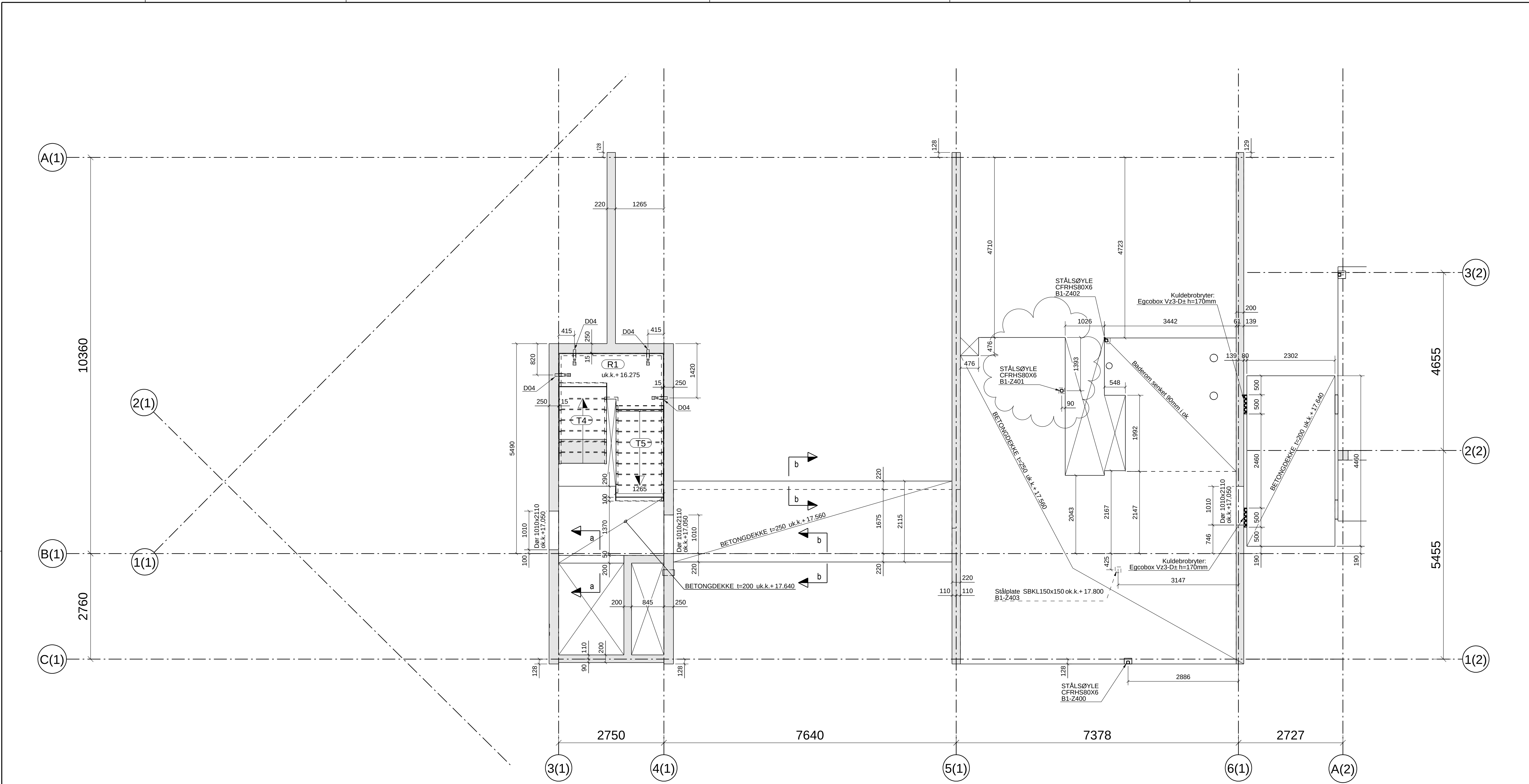
Bygg 1 PLAN +17.84
