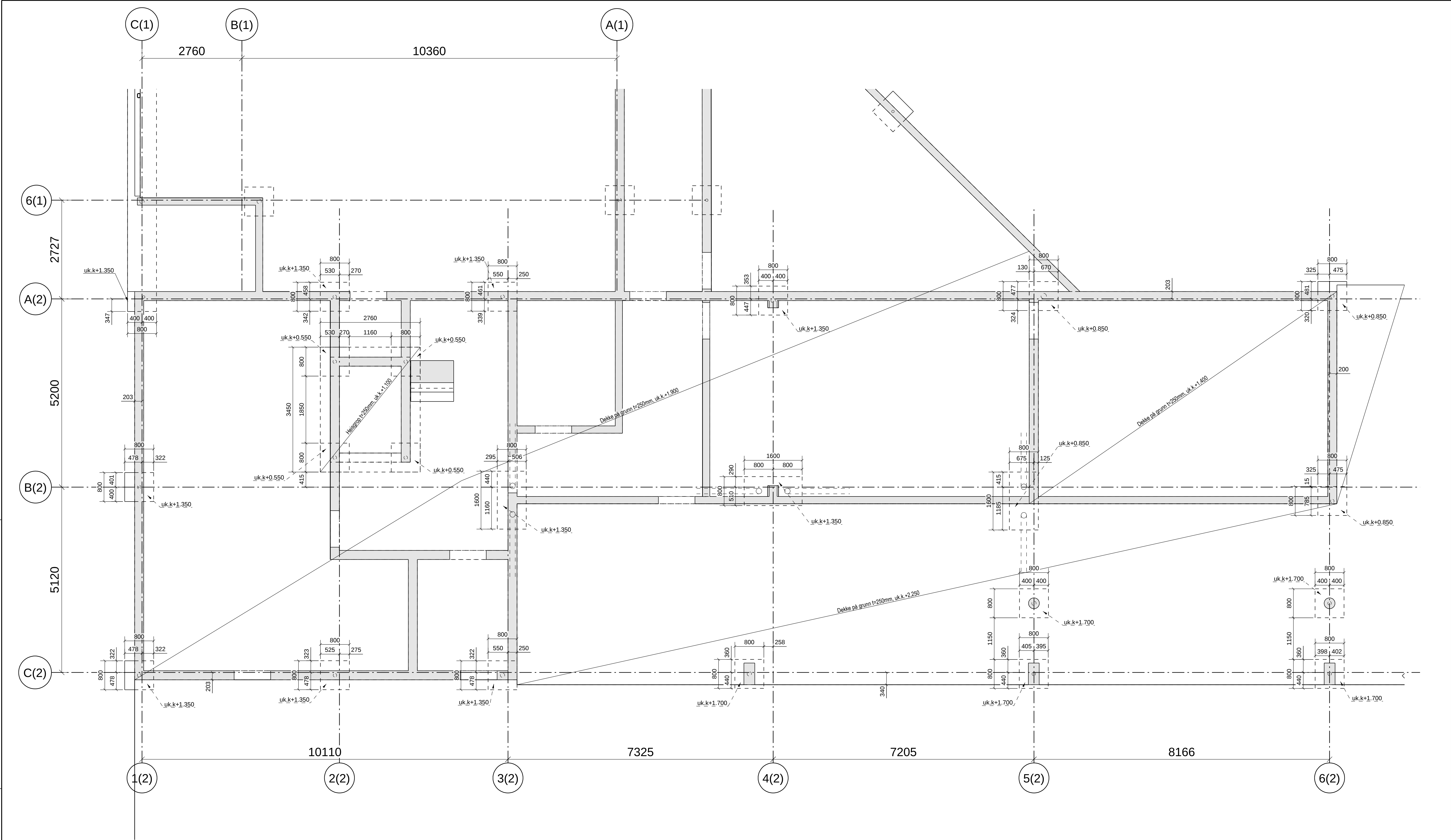
Bygg 2 PLAN +2.50
