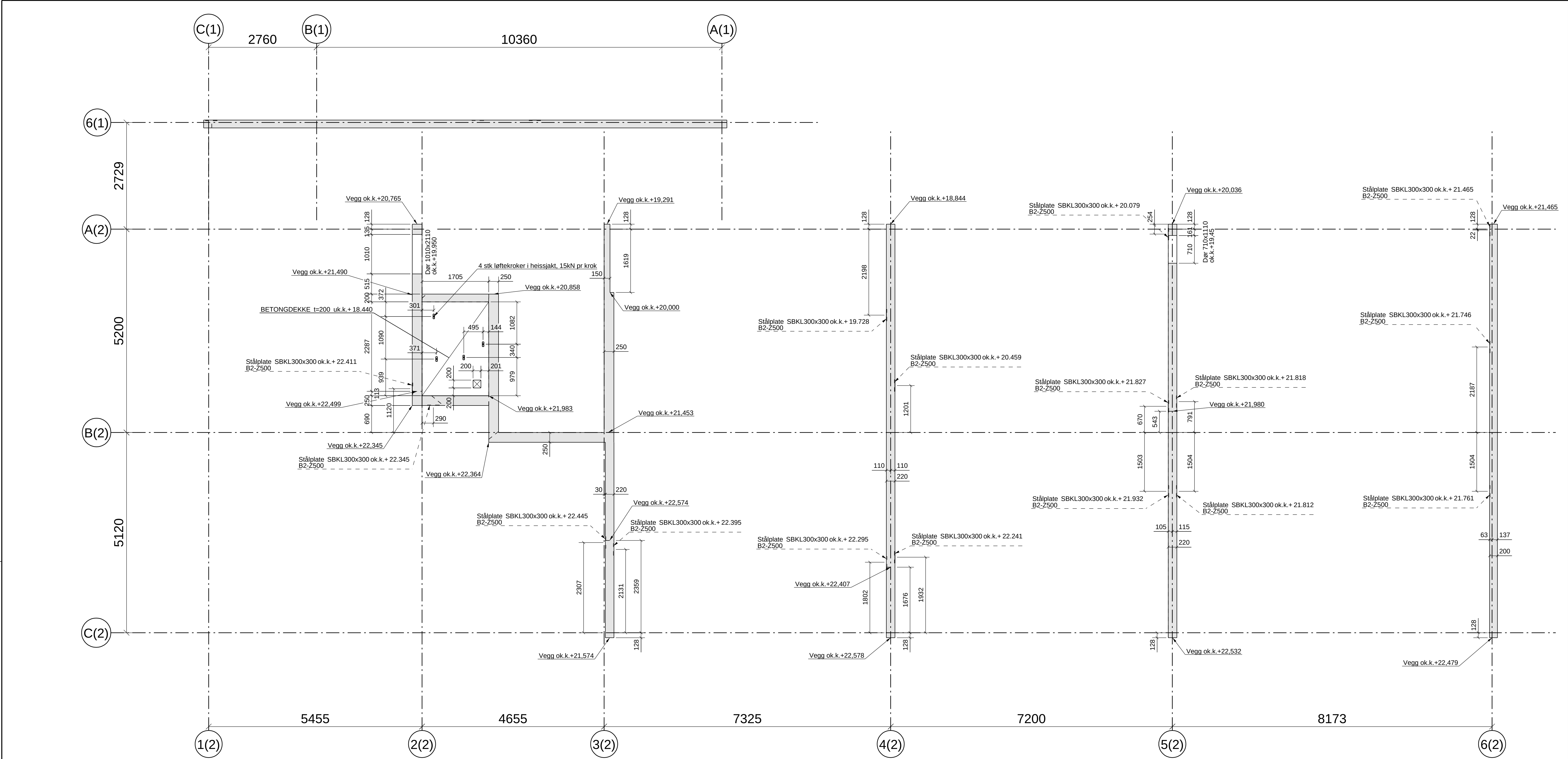
Bygg 2 PLAN +20,74
