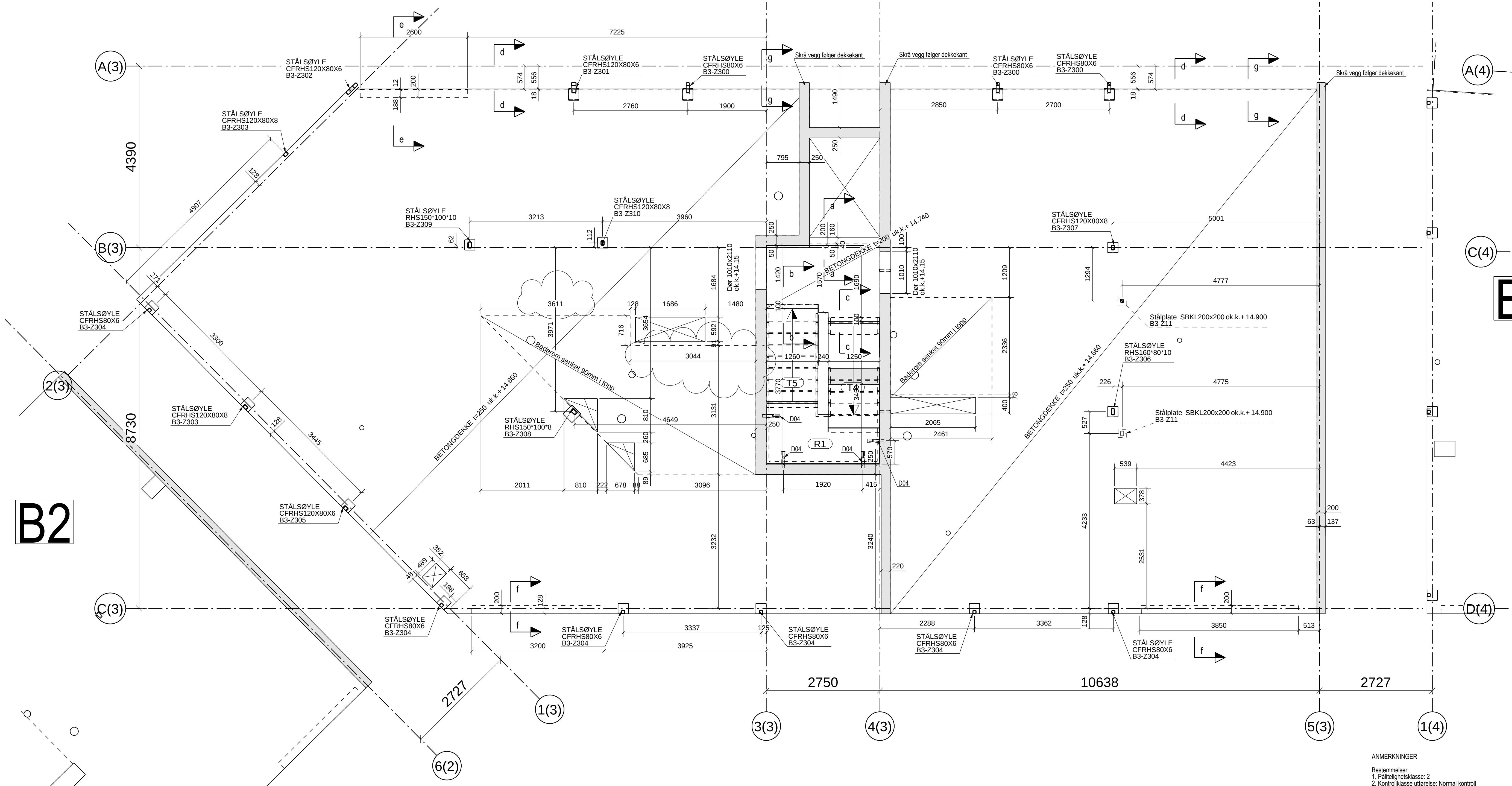
Bygg 3 PLAN +14.94
