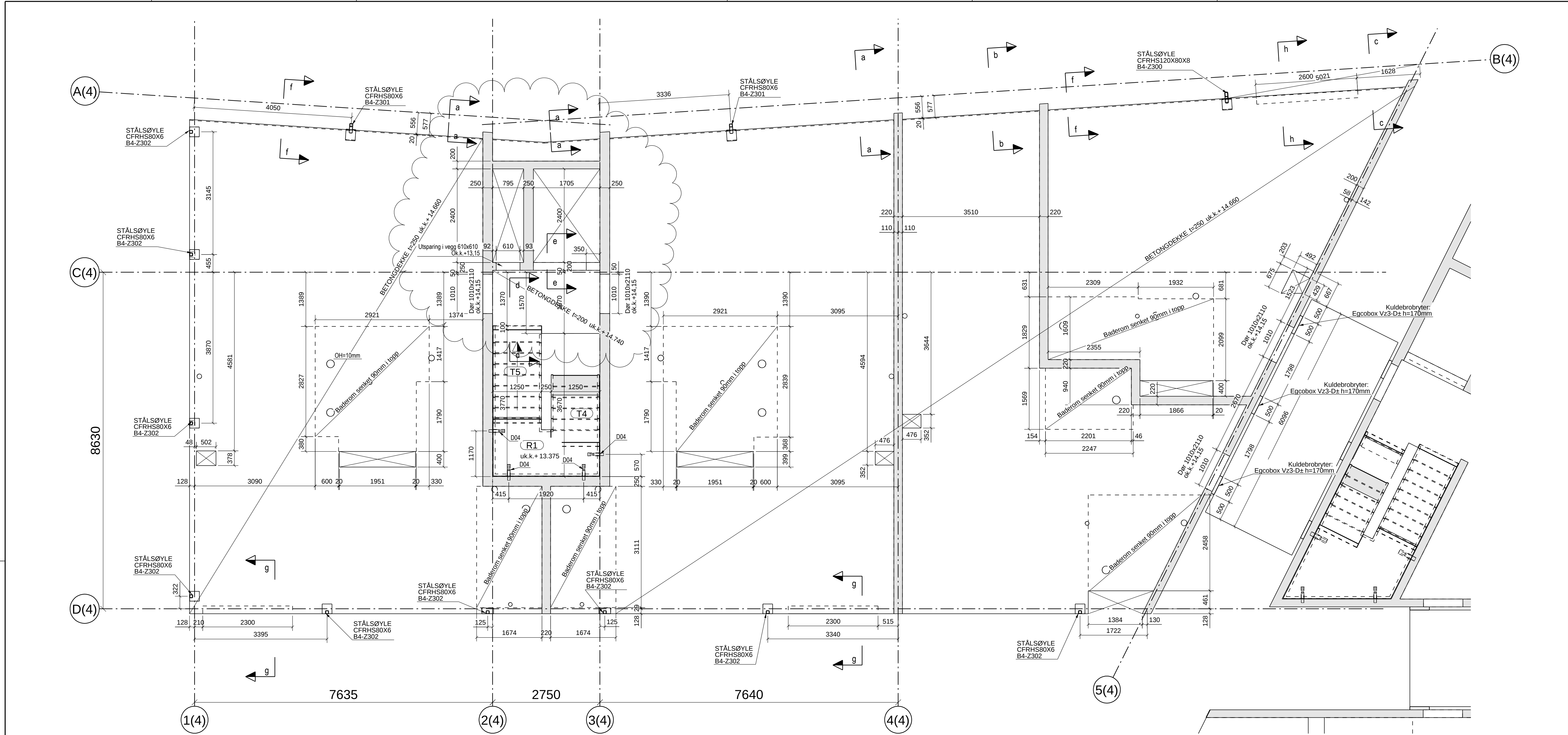
Bygg 4 PLAN +14.94
