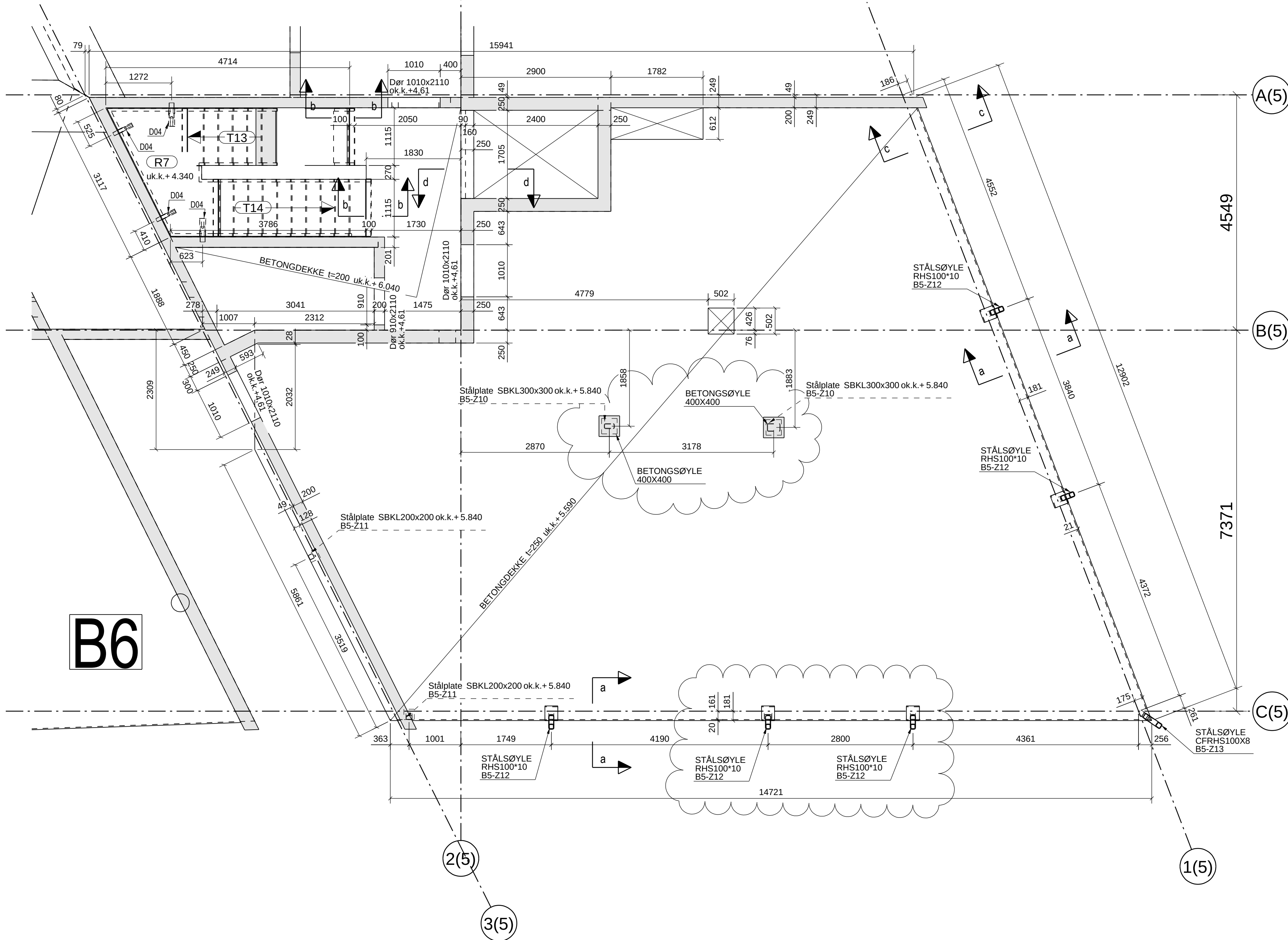
Bygg 5 PLAN +6.24
