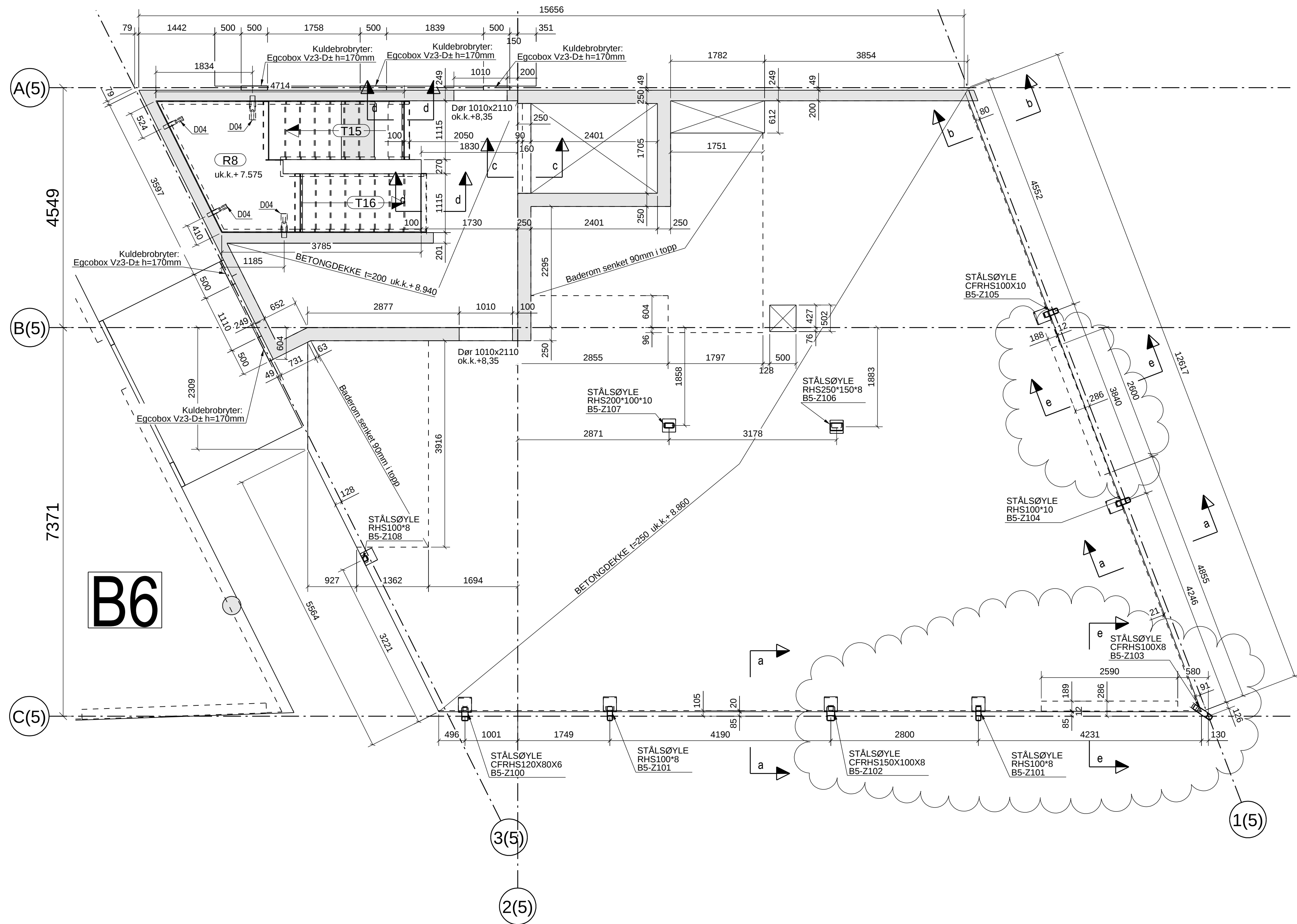
Bygg 5 PLAN +9.14
