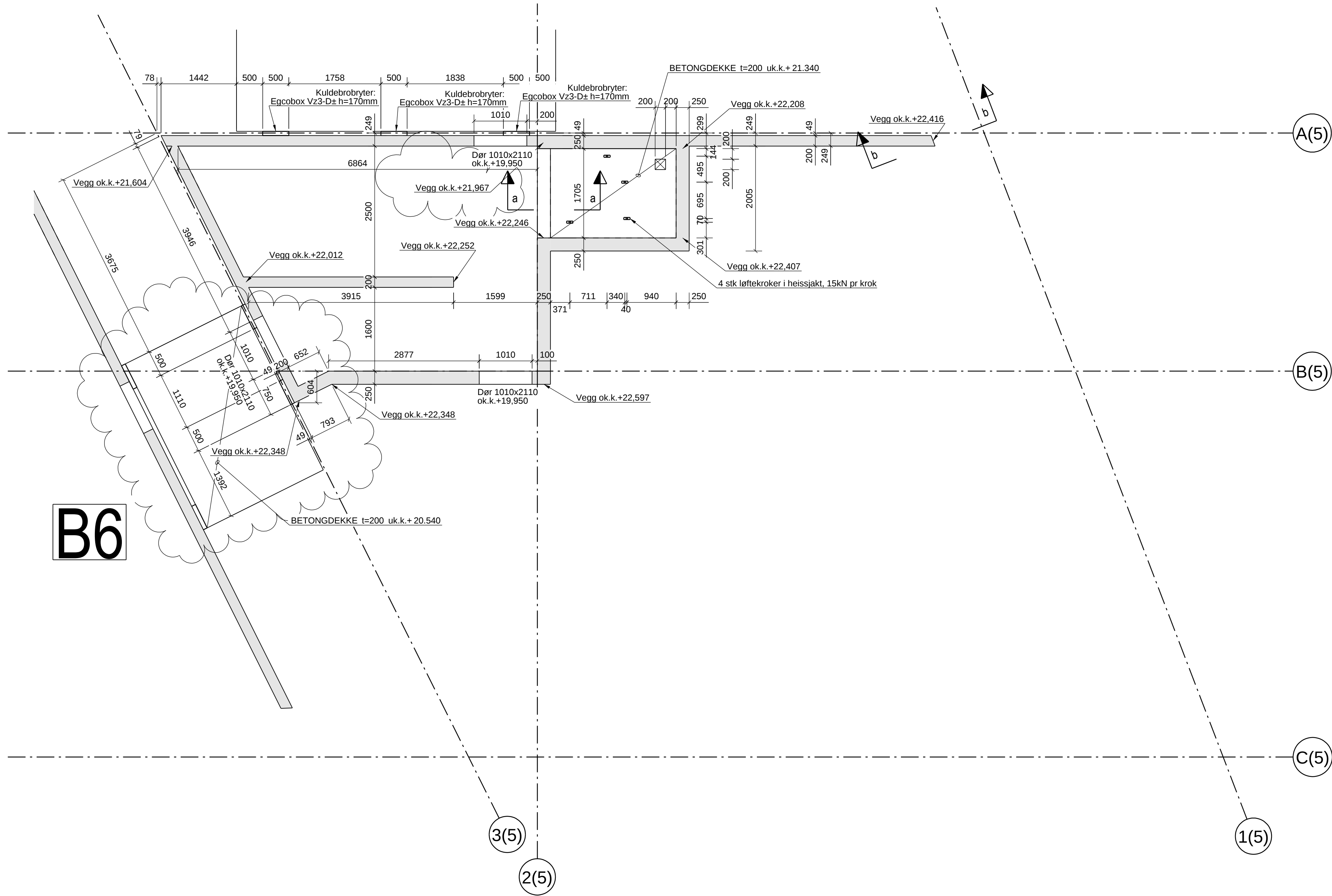
Bygg 5 PLAN +20.74
