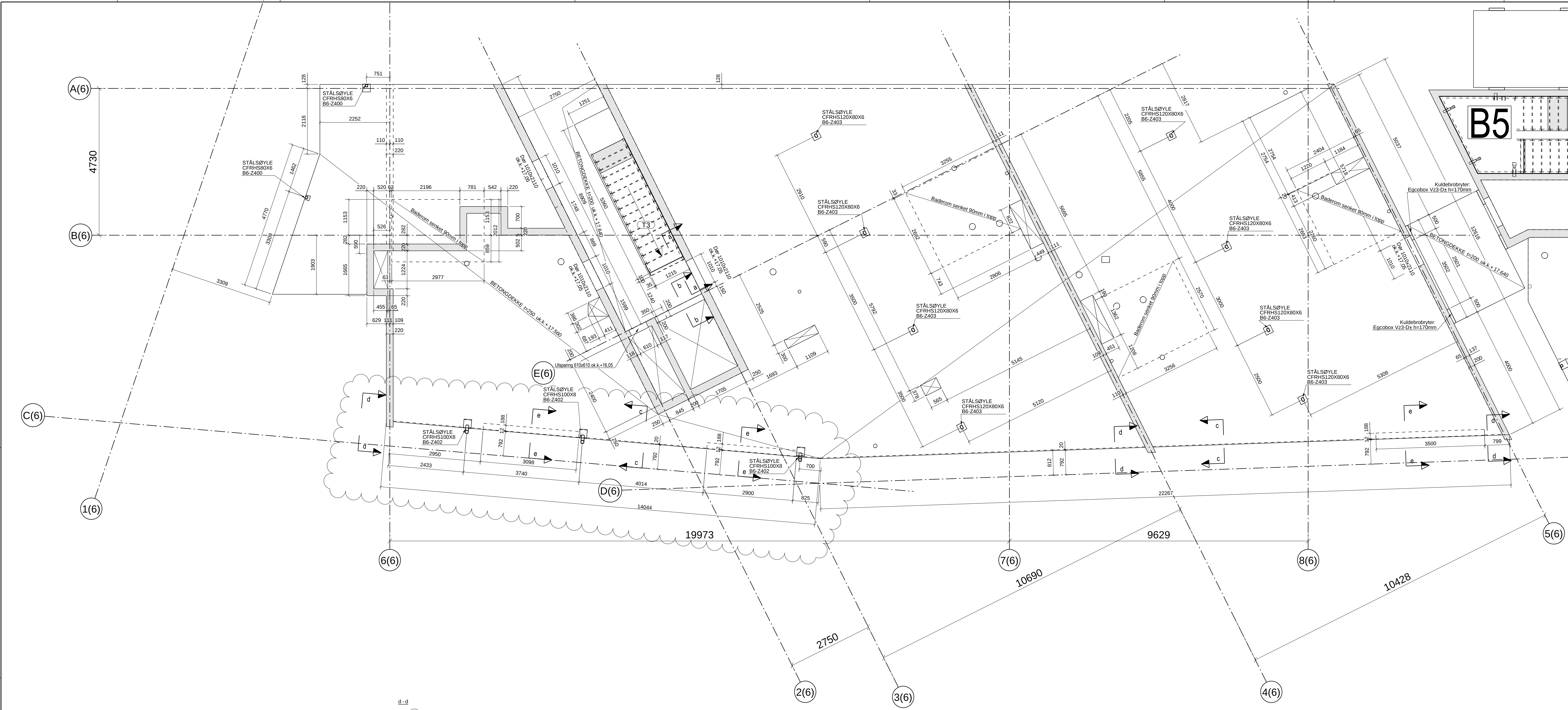
Bygg 5 PLAN +17.84
